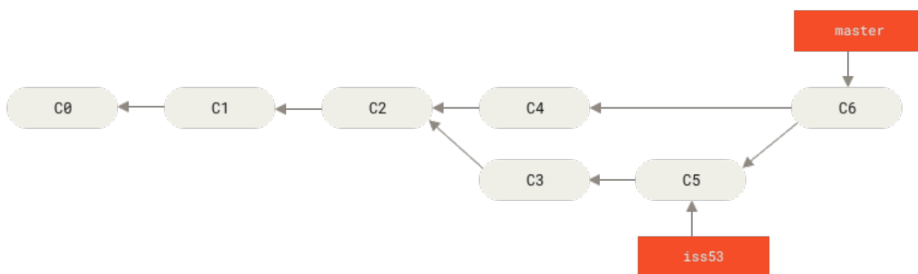
Рисунок 25. Коммит слияния
